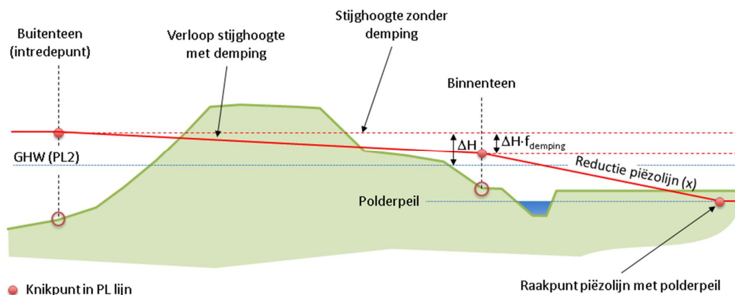
Figuur 4.3 Gebruik van dempingsfactor ( f ) en reductie piëzoliijn aan de polderzijde ( X ) voor schematisering horizontaal stijghoogte verloop
