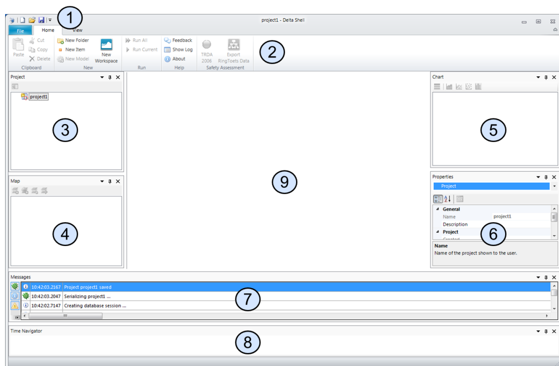
Figuur 3.3: De WTI interface
